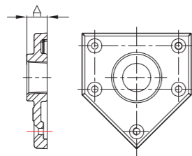
Tee Flange
